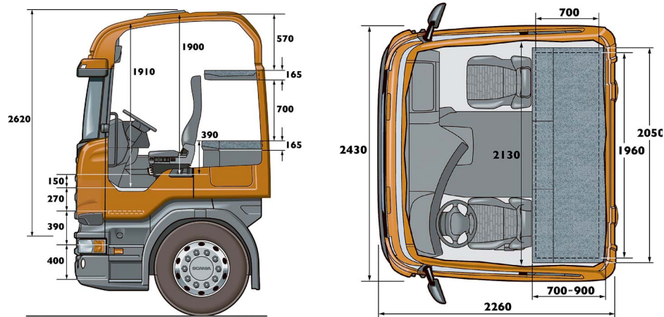
Чертеж кабины
